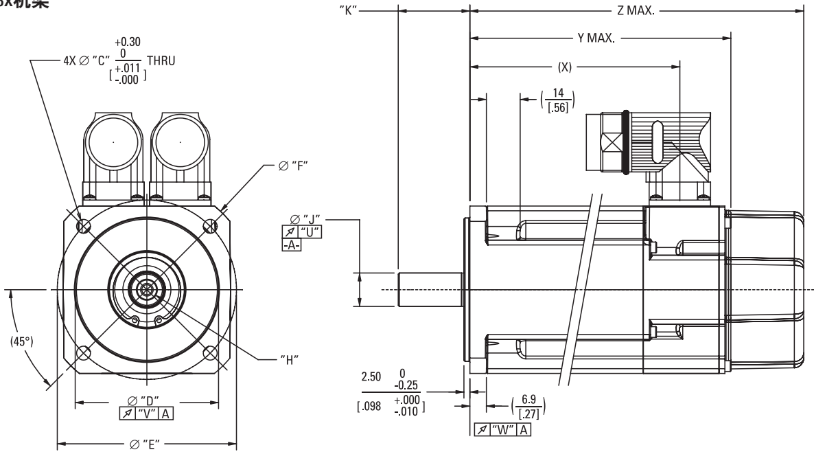
AKM3x机架
