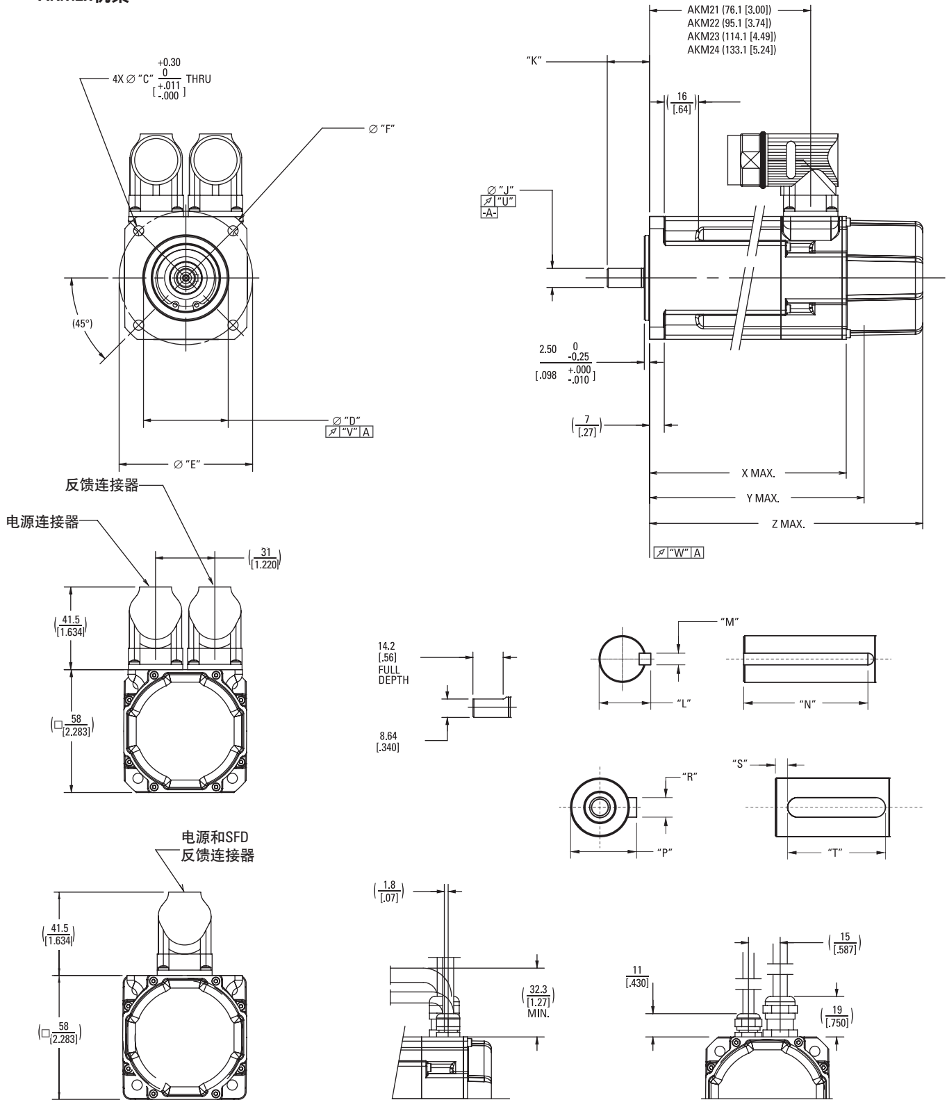
AKM2x机架
