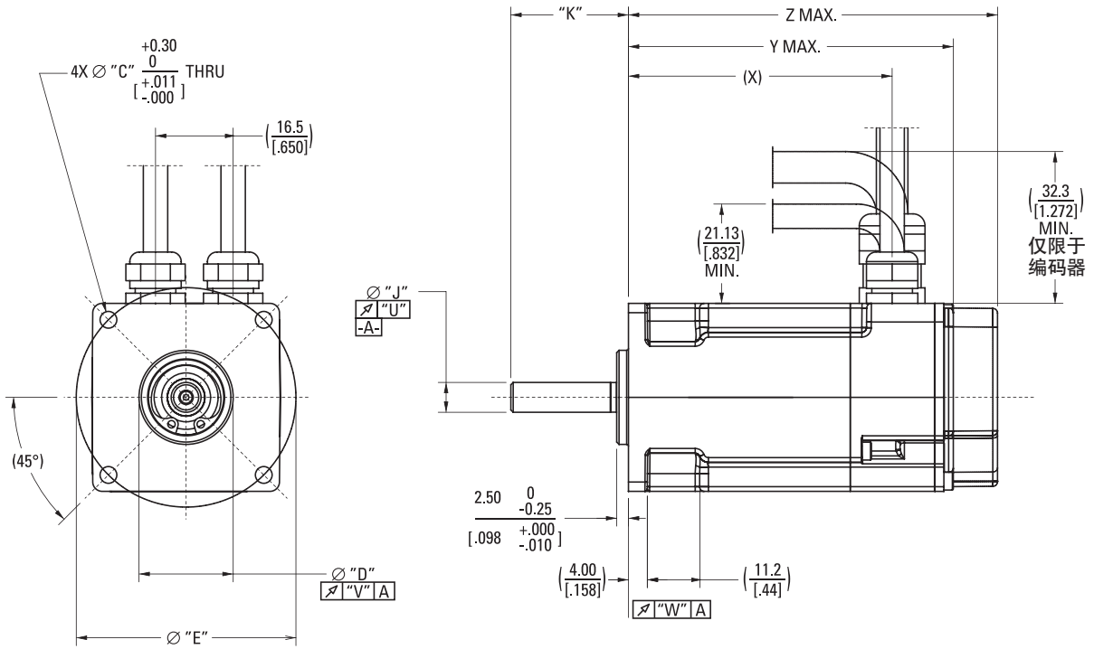
AKM1x机架
