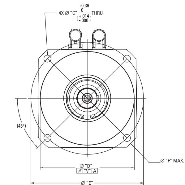
AKM7x机架
